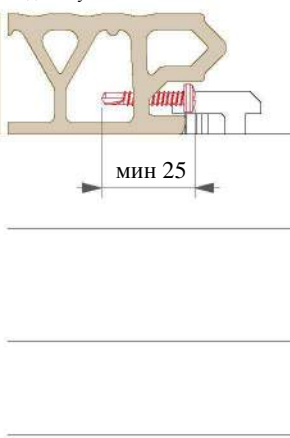
вид сбоку
